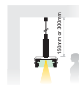
PENDANT Installation
