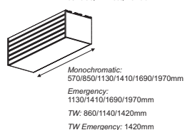
Surface, Trimless, Pendant
